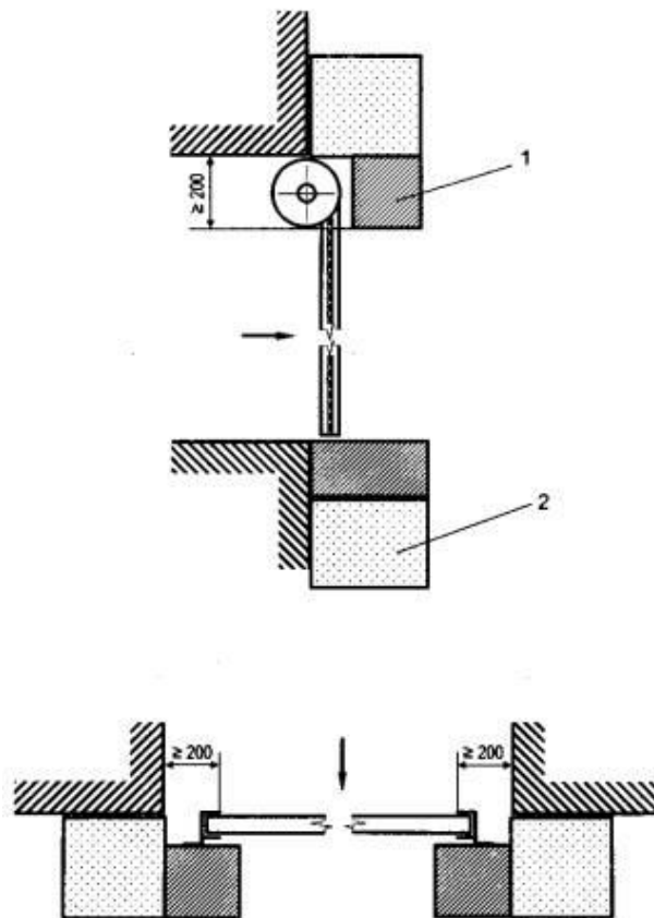
1 - фрагмент ограждающей конструкции; 2 - рама для установки фрагмента ограждающей конструкции; →, ↓ - направление теплового воздействия
