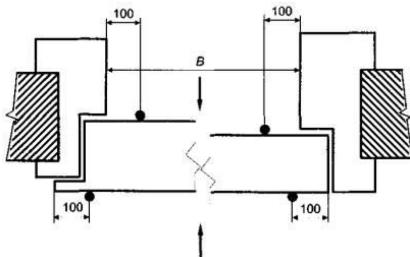
Рисунок 12 - Схема установки термодпар на необогреваемой поверхности полотна распашной однопольной двери в зоне 100 мм от его торцевых поверхностей и проема в свету (горизонтальное сечение)
