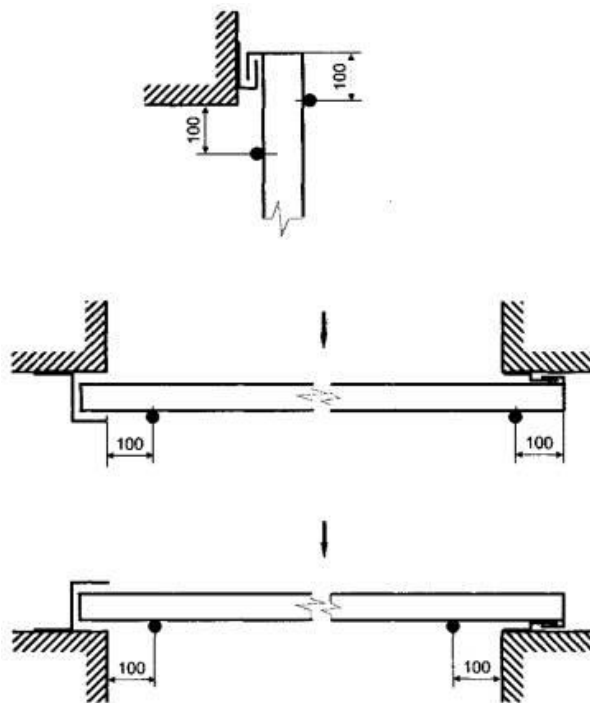
Рисунок 14 - Схема установки термодпар на необогреваемой поверхности полотна откатной двери (ворот)
