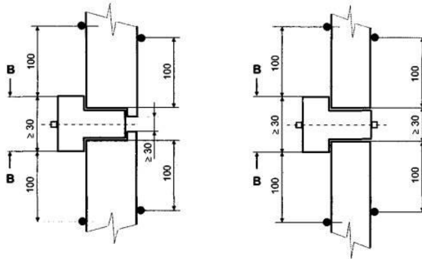
Рисунок 20 - Схема установки термодатчика на необогреваемой поверхности распашной двупольной двери с фрамугой в зоне 100 мм от торцевых поверхностей коробки (вертикальное сечение)
