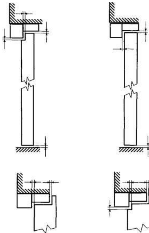
Рисунок 25 - Примеры замеров зазоров распашных дверей (горизонтальное сечение)
