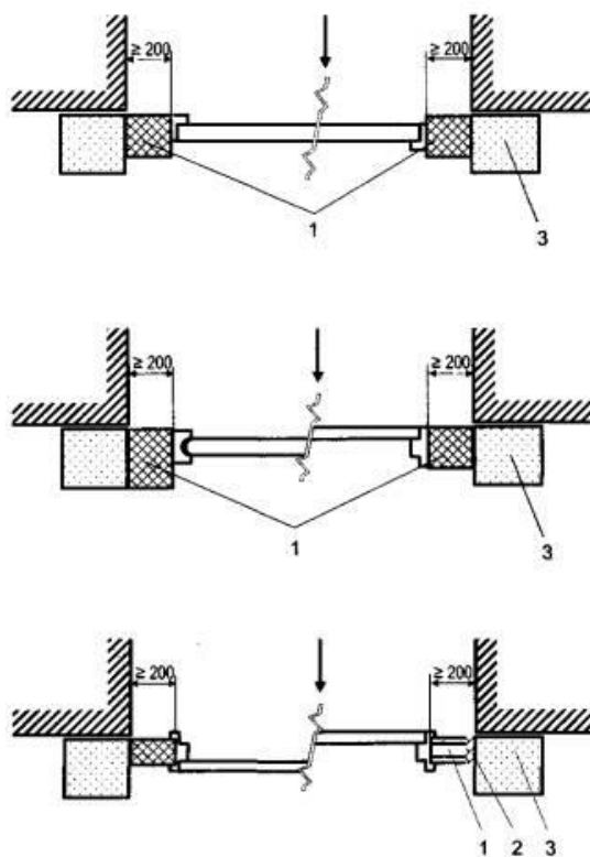
1 - фрагмент ограждающей конструкции; 2 - теплоизоляционная прокладка; 3 - рама для установки фрагмента ограждающей конструкции; ↓ - направление теплового воздействия
