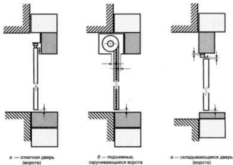
Рисунок 27 - Примеры замеров зазоров (вертикальное сечение)
