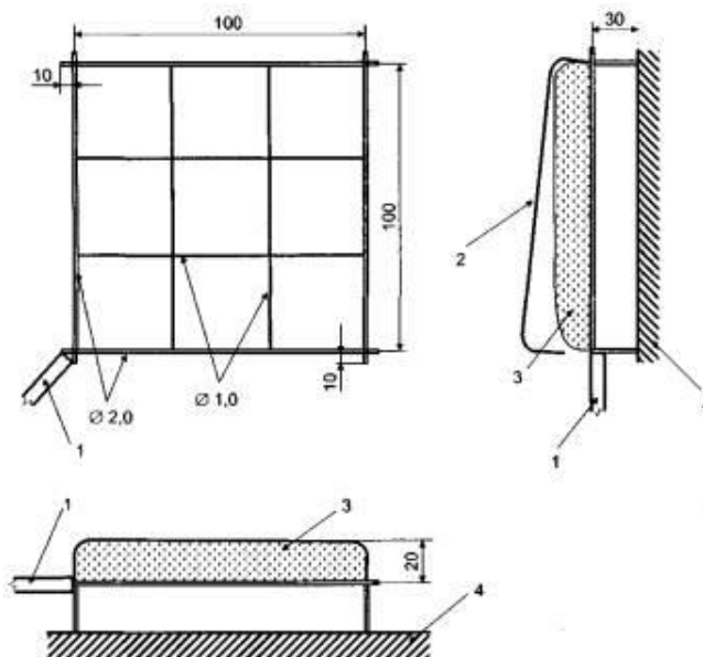
Рисунок 28 - Рамка для закрепления ватного тампона
