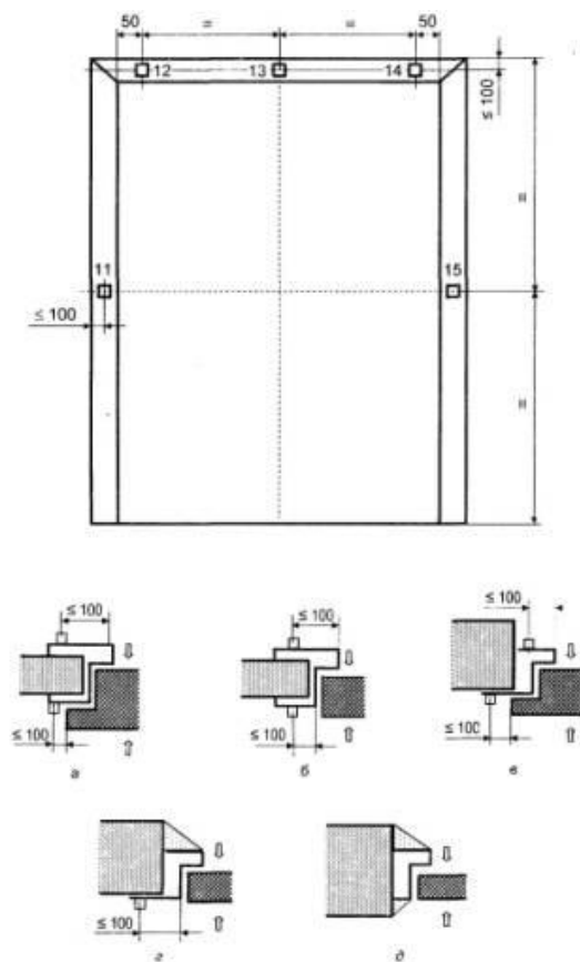
Рисунок 16 - Схема установки термопар на необогреваемых поверхностях полотен подъемных и скручивающихся ворот
